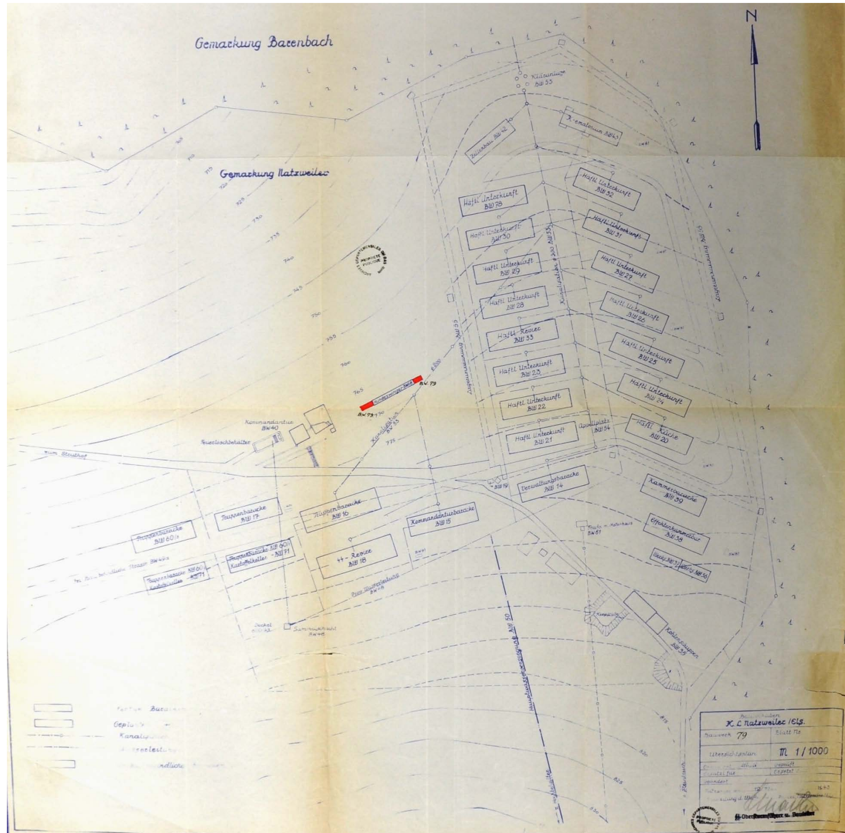
Echelle : 1:1000 e , 59 cm x 61,8 cm
